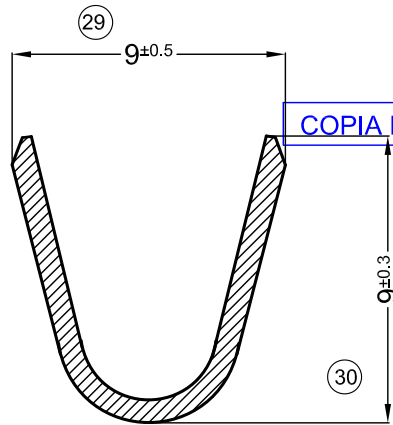
SECC. B-B
