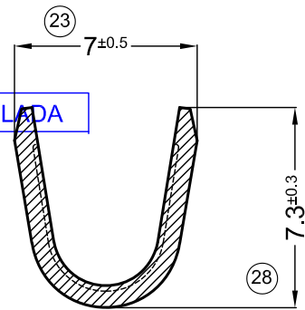
SECC. A-A
